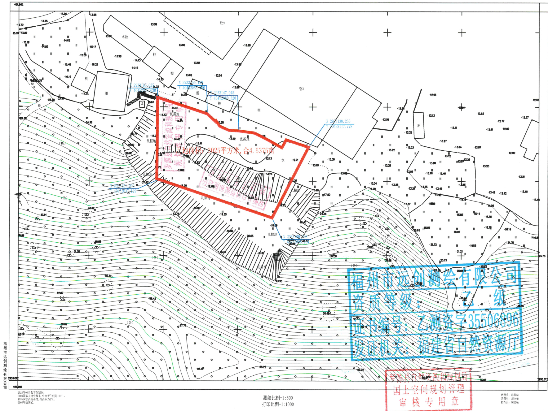
起步镇上长治村何处肥片区锦源纺织周边配套设施（排水项目）用地红线图
