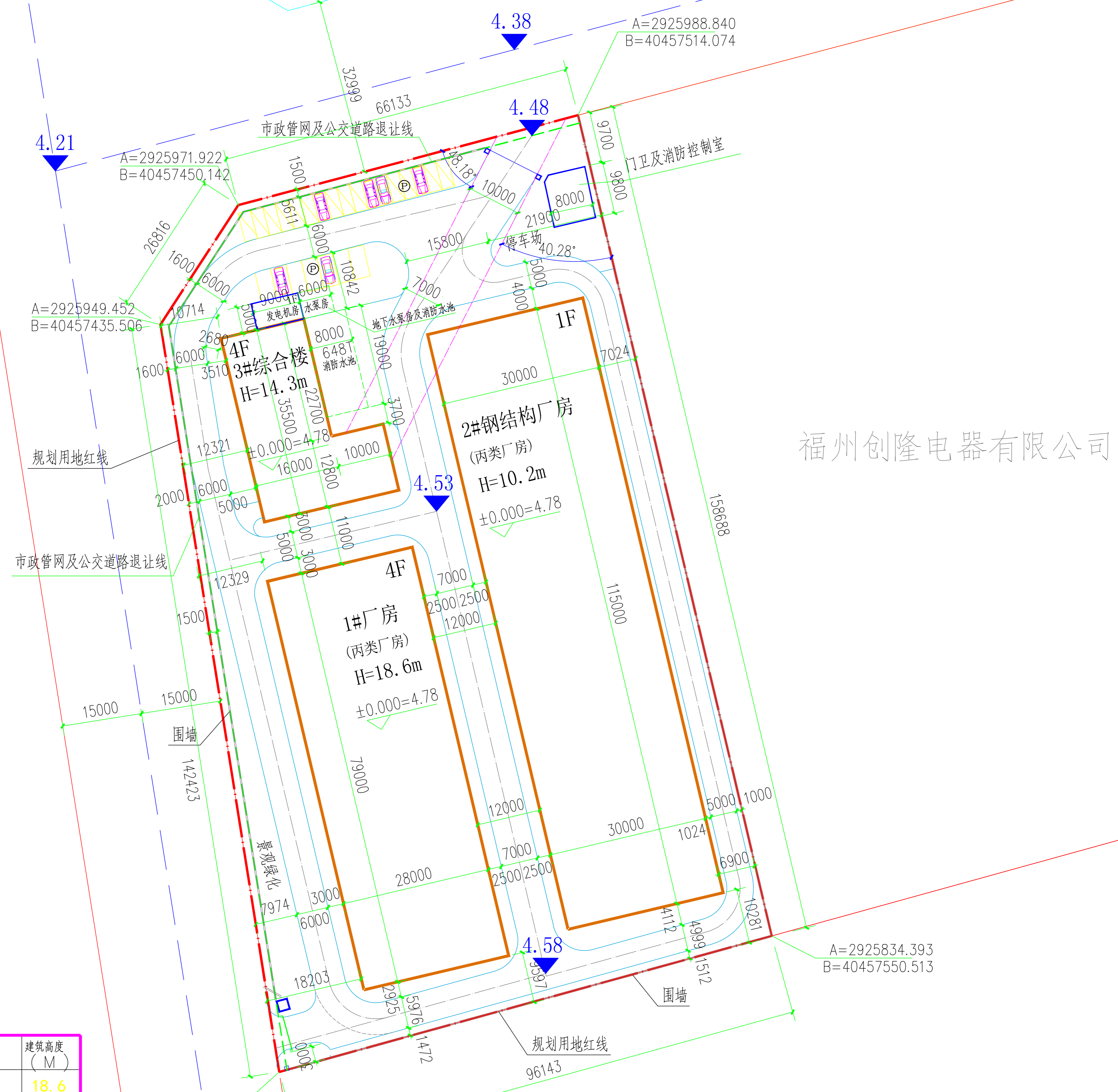
总平面图 1:500
