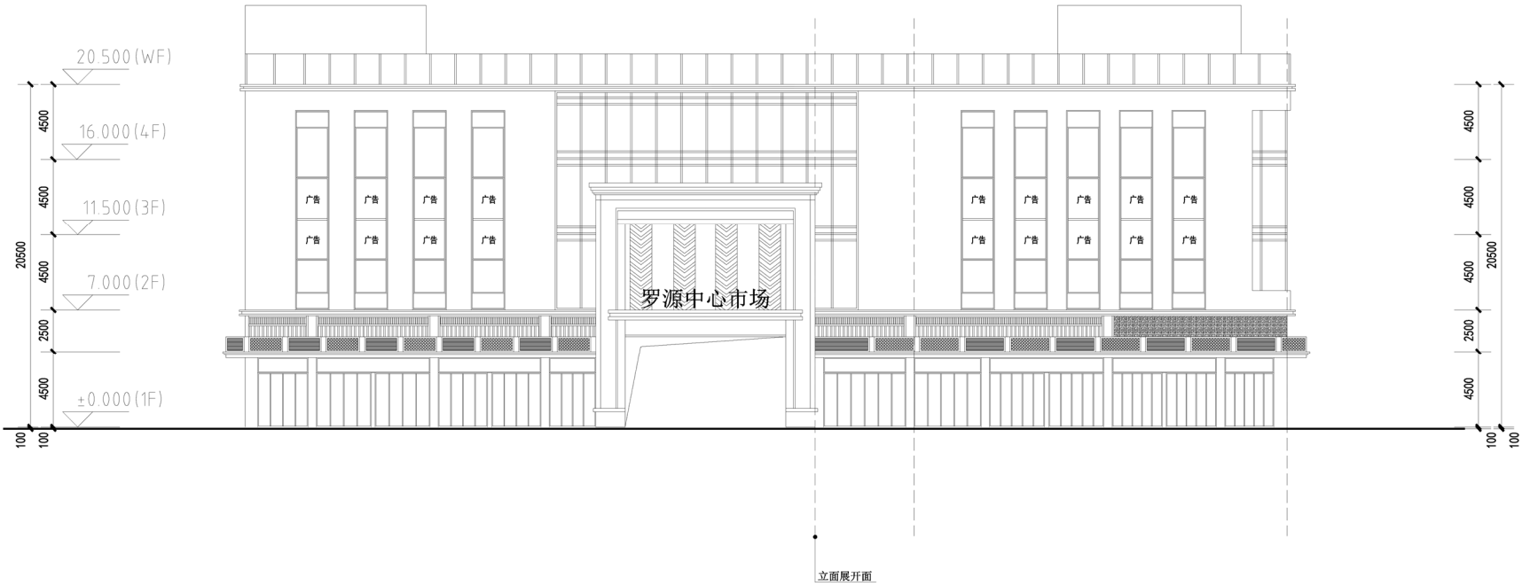
中心市场西立面
