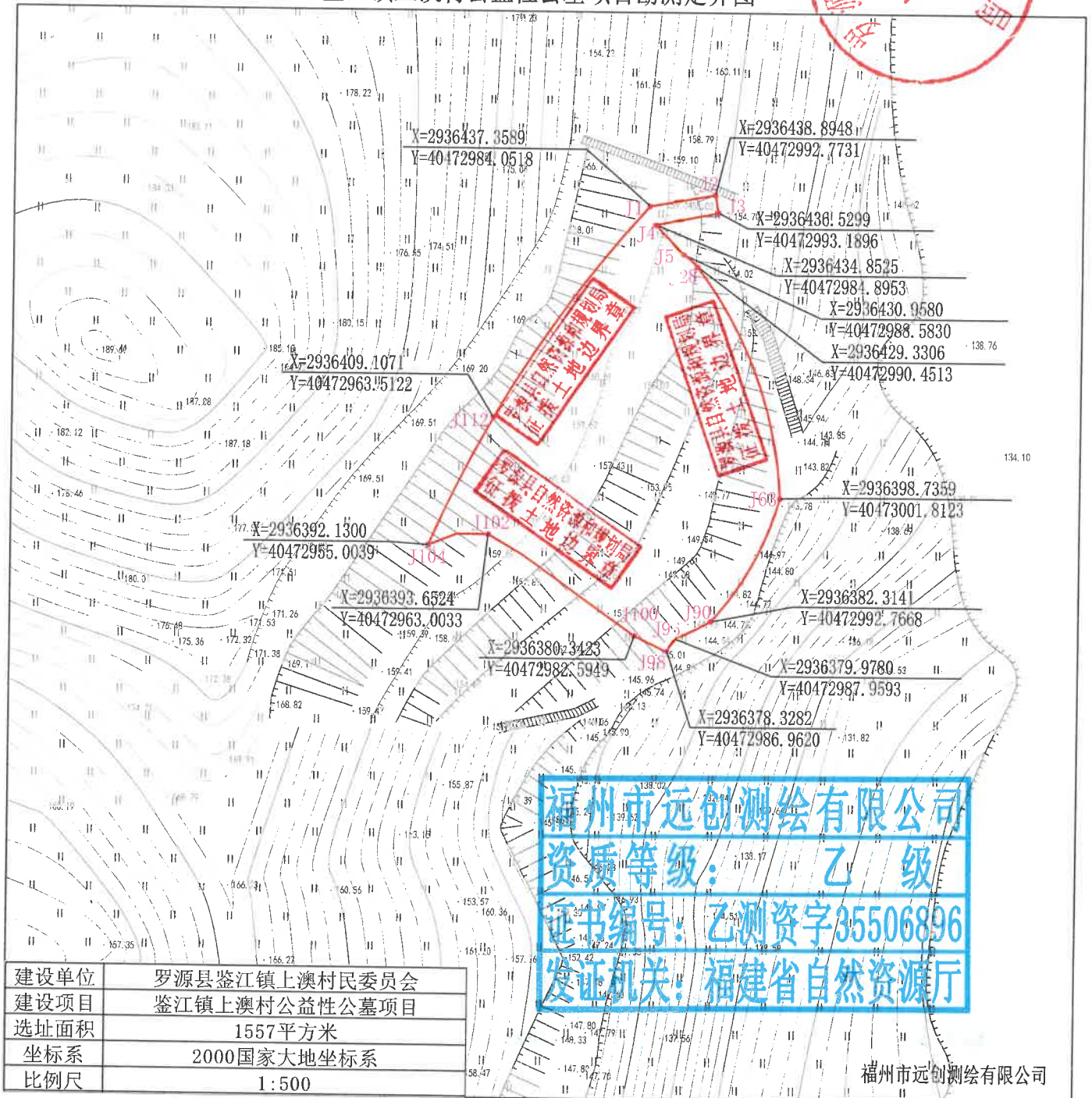
鉴江镇上澳村公益性公墓项目勘测定界图
